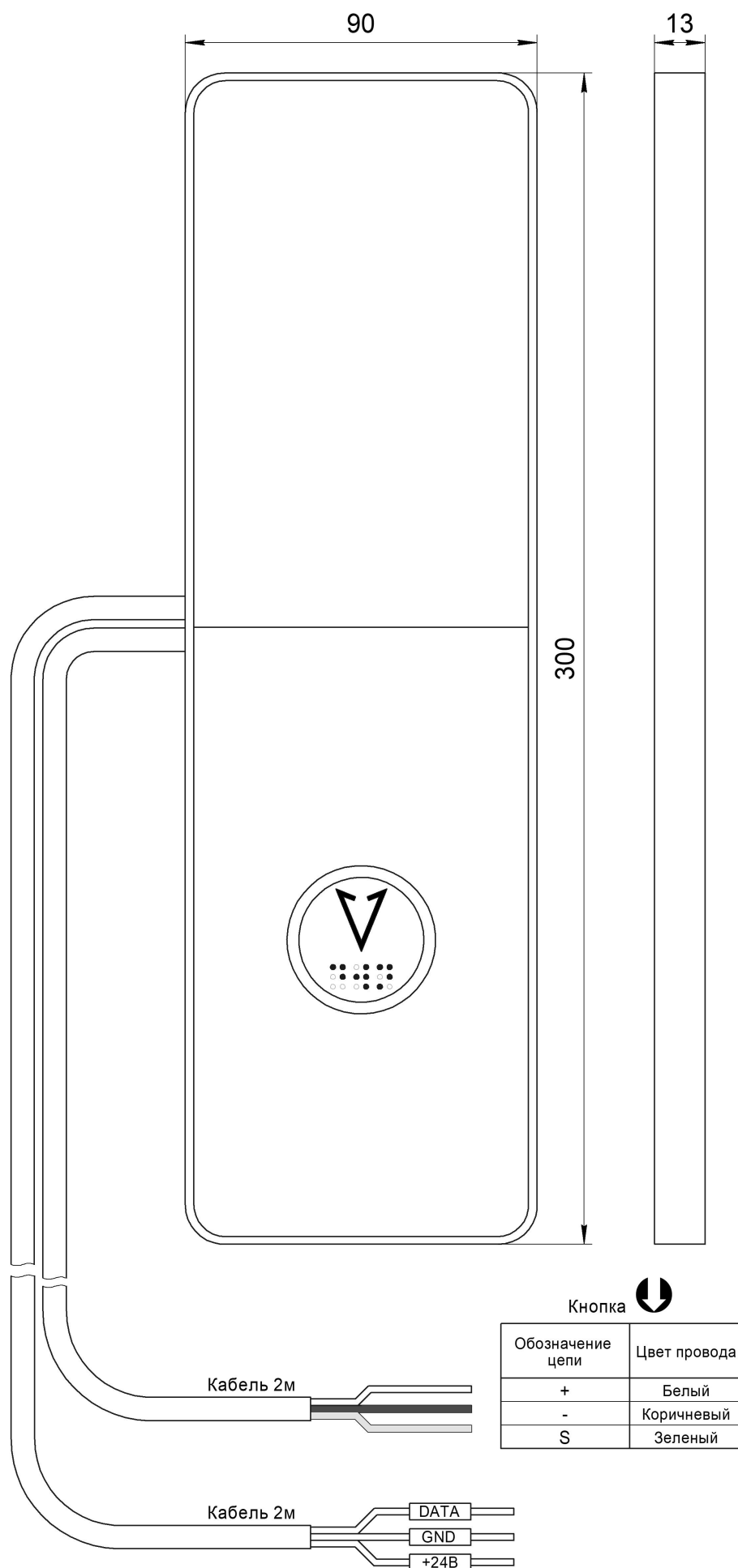
Рис.1 Внешний вид Вызывной пост ОНИКС НШЕК.468381.027-01
